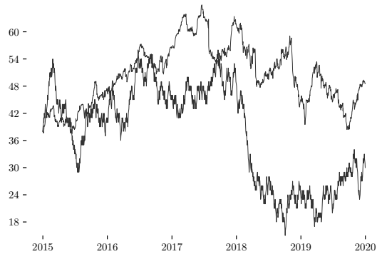
153: Altria & Coin Tosses
